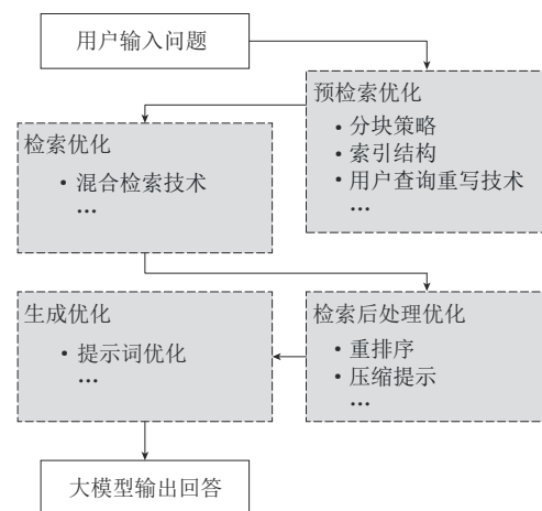
图3 RAG流程改进框架
